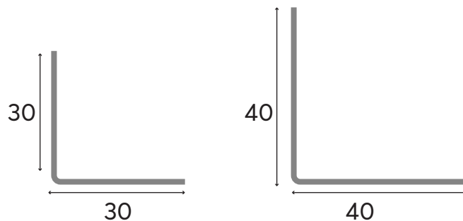
Mặt cắt cột V
